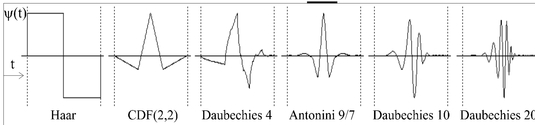
Príklady rôznych druhov základných waveletov
