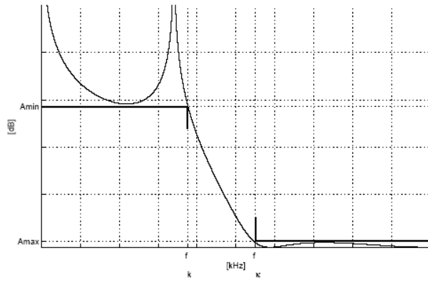
Frekvenčná charakteristika prevádzkového tlmenia
